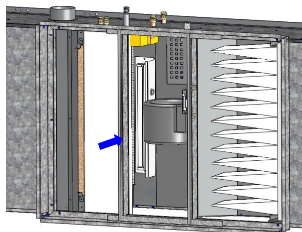
Lâmpada UV. (opcional)
