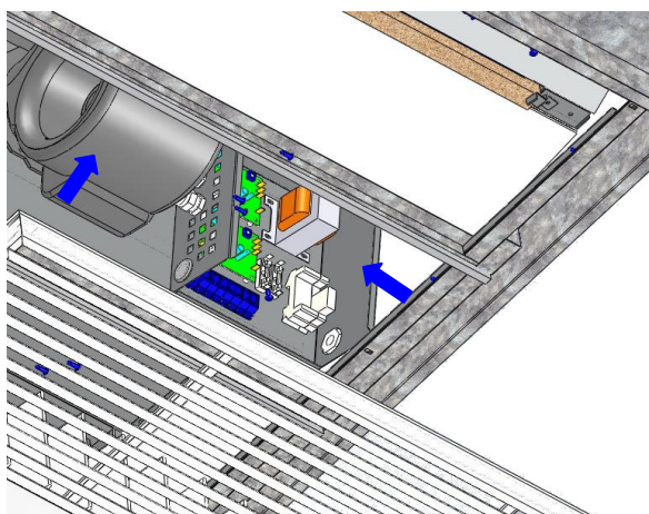
Painel Elétrico e ventilador
